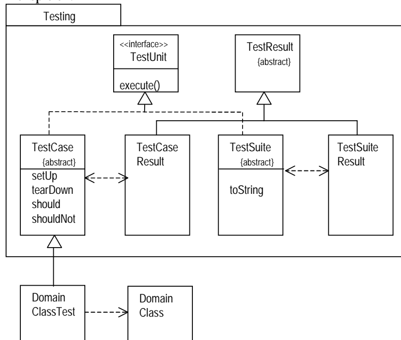
Abbildung 5: Aufbau des Test-Frameworks
