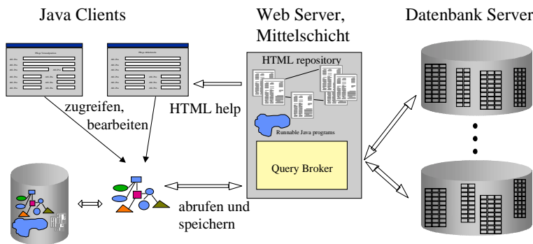
Abbildung: 2: Adaptierte Dreischichten-Architektur
