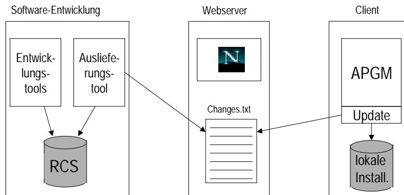
Abbildung 3: Integration von automatischem Update und Softwareentwicklung
