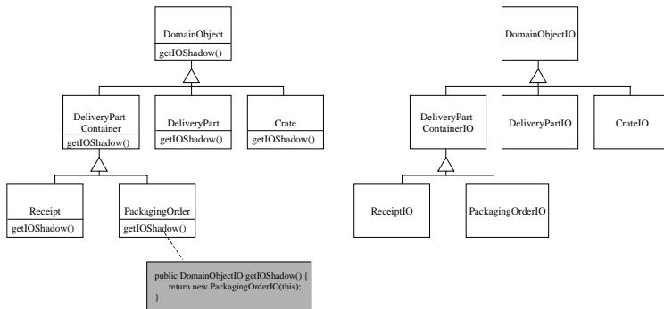
Abbildung 4: Schattenhierarchie-Muster
