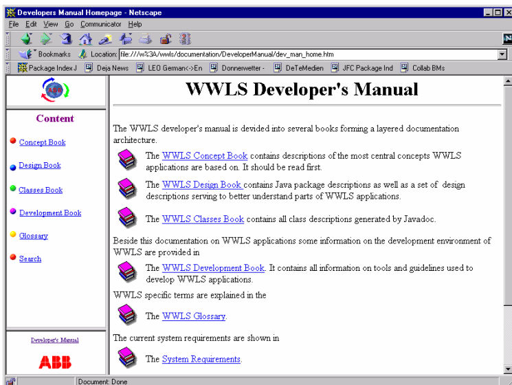
Abbildung 6: Das WWLS-Dokumentationssystem
